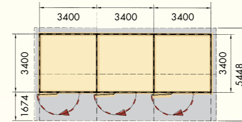
3 Die Reihenboxen erlauben eine beliebige Erweiterung.
