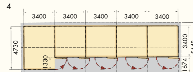
4 Die Kopfbox am Ende einer Reihe bietet sich auch als Lager oder Sattelkammer an.
